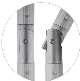
Automatische Knickfunktion
